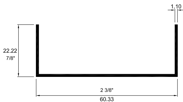
7839 CANAL
