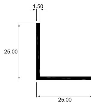
4110 ÁNGULO IGUAL
