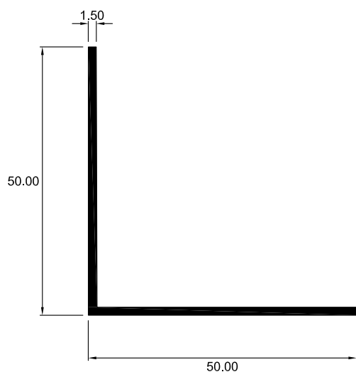
4320 ÁNGULO IGUAL
