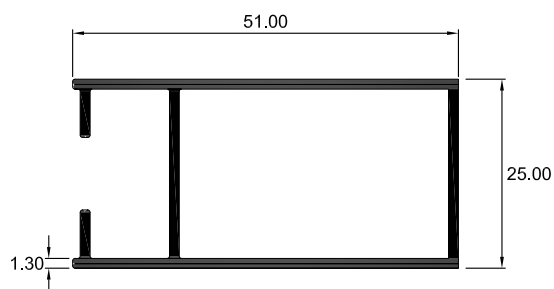
2510 PIERNA
