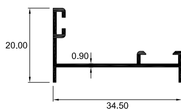
7311 PORTA JUNQUILLO
