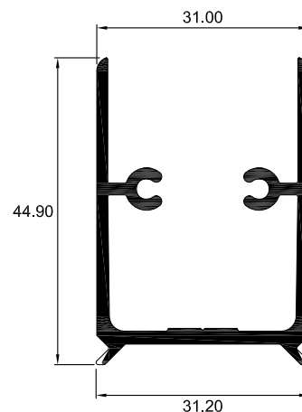
3511 ESPIGA S-35
