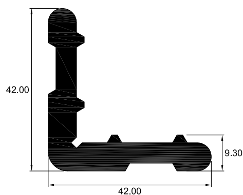
3805 ESPIGA
