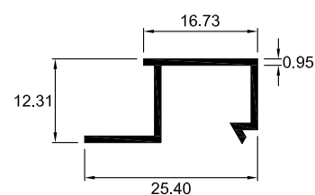
7305 JUNQUILLO
