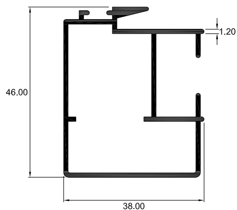
2511 TRASLAPO REFORZADO
