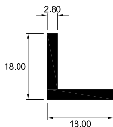
4016 ÁNGULO IGUAL
