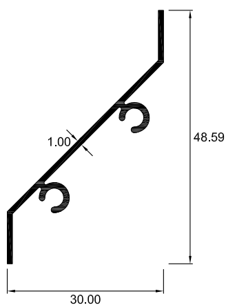
0315 QUIEBRAVISTA
