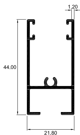
2504 CABEZAL
