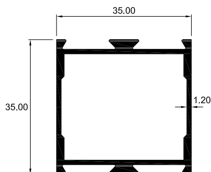
3508 BASTIDOR
