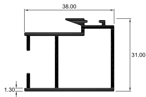
2507 TRASLAPO
