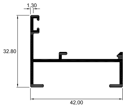
4201 MARCO
