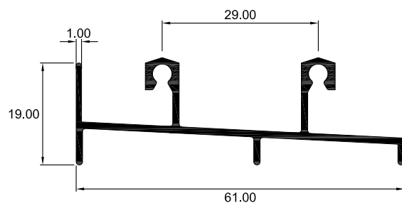
2002 RIEL INFERIOR
