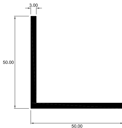
4020 ÁNGULO IGUAL
