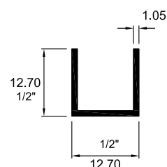
3004 CANAL DE 1/2"
