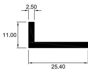
4011 ÁNGULO DESIGUAL
