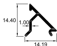
3503 JUNQUILLO 45°
