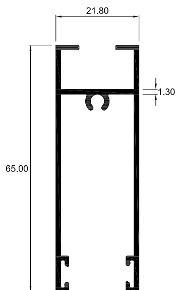
2505 ZÓCALO
