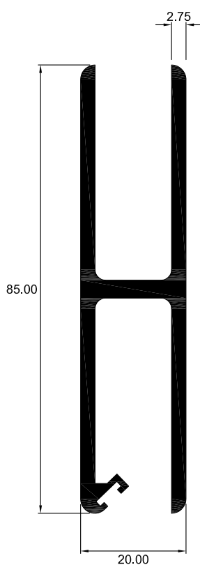
7902 Nombre: ZÓCALO
