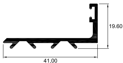
3509 TRASLAPO
