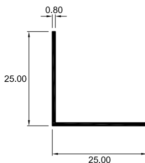
4109 ÁNGULO IGUAL
