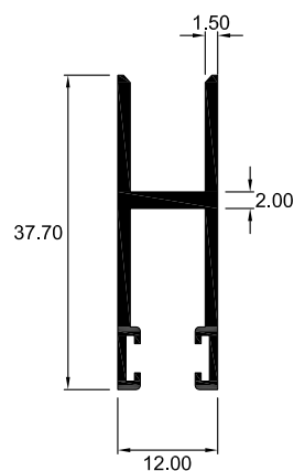
8224 ZÓCALO
