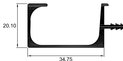
2013 TIRADOR
