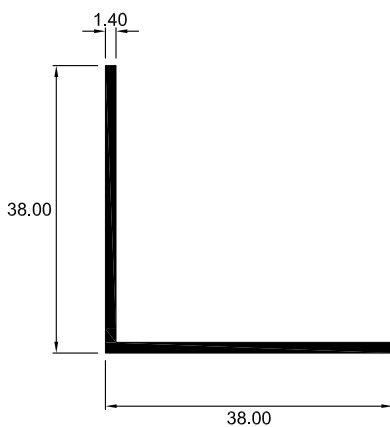
4314 ÁNGULO IGUAL
