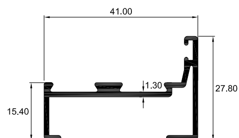
3502 MARCO
