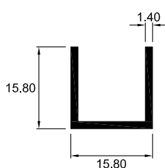
3014 CANAL
