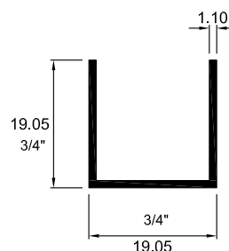
3007 CANAL DE 3/4"
