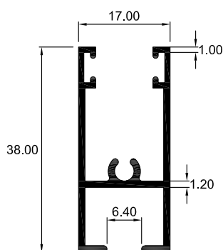
2004 CABEZAL
