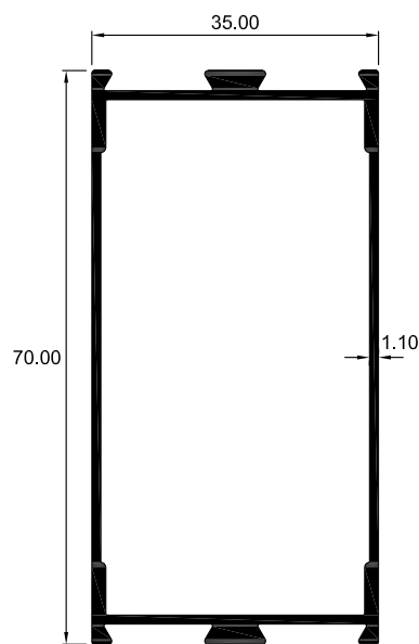
3501 BASTIDOR
