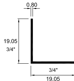
4108 ÁNGULO IGUAL
