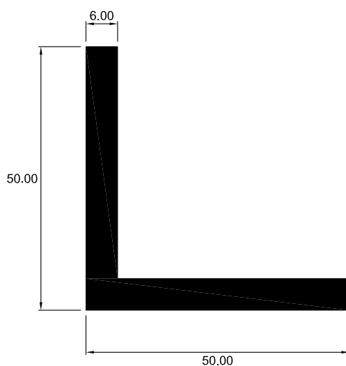
4322 ÁNGULO IGUAL
