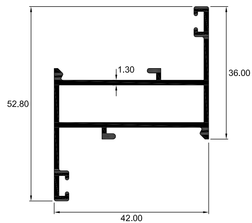
4202 HOJA
