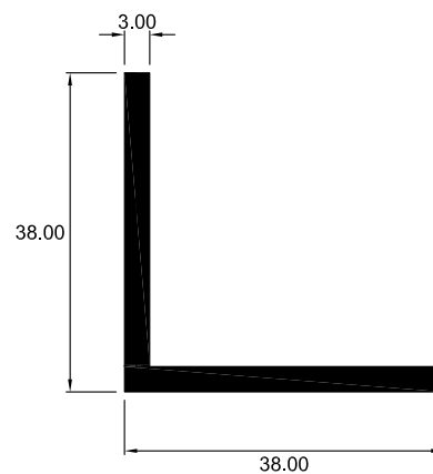
4012 ÁNGULO IGUAL
