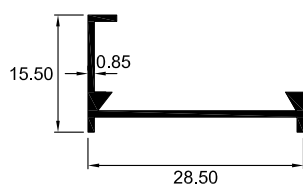
7300 PORTAJUNQUILLO
