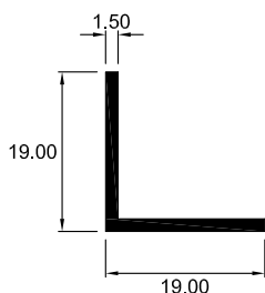
4107 ÁNGULO IGUAL
