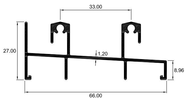
2502 RIEL INFERIOR
