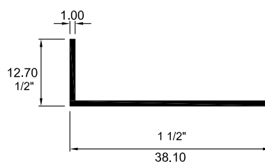
4013 ÁNGULO DESIGUAL
