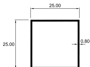
5331 TUBO CUADRADO
