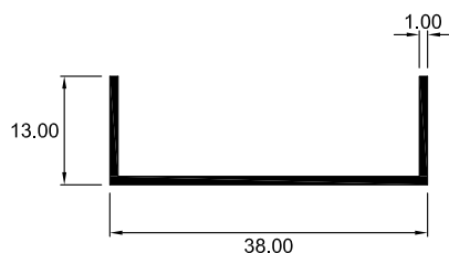
3313 CANAL
