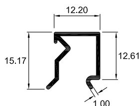
3512 JUNQUILLO RECTO
