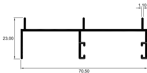
2509 JAMBA
