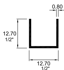
3002 CANAL
