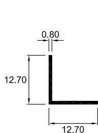
4102 ÁNGULO IGUAL
