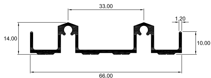
2503 RIEL INFERIOR
