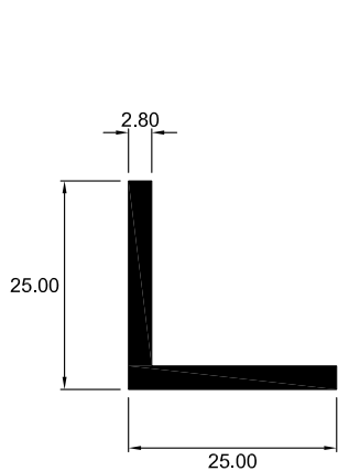
4009 ÁNGULO IGUAL
