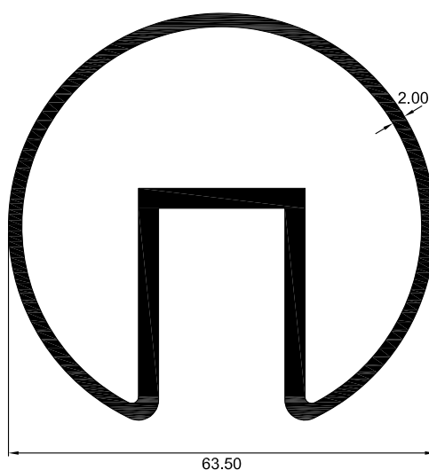
2603 PASAMANOS CIRCULAR
