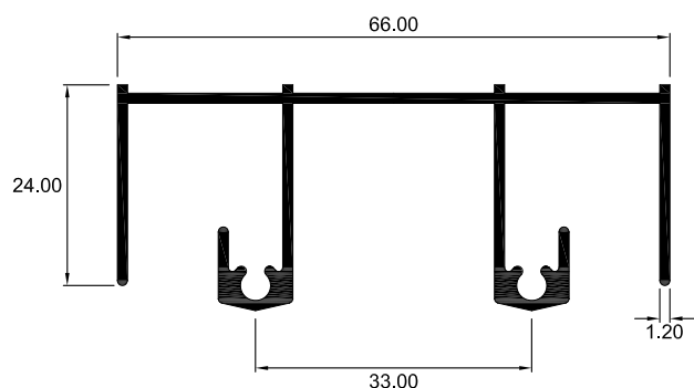
2501 RIEL SUPERIOR
