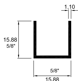
3011 CANAL DE 5/8"
