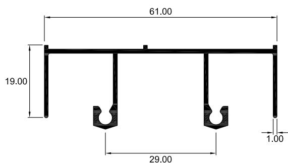
2001 RIEL SUPERIOR
